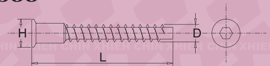
A0355 D*L*H
