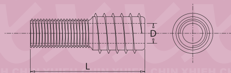
A1012 D*L
