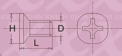
A0371 D*L*H
