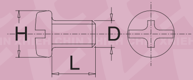
A0353 D*L*H
