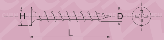
B0359 D*L*H
