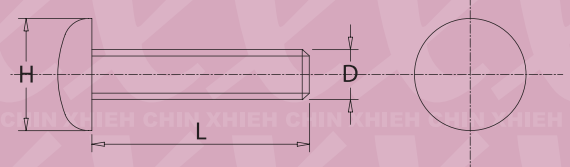
A1041 D*L*H
