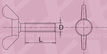
A0351 D*L
