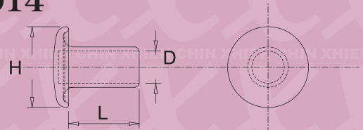
A1014 D*L*H
