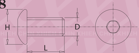
A1028 D*L*H
