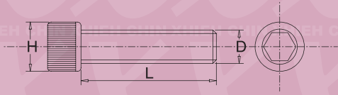
A0335 D*L*H
