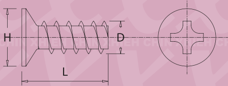
A1043 D*L*H
