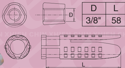
A1047 D*L
