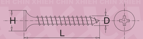
B0361 D*L*H
