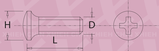
A0367 D*L*H
