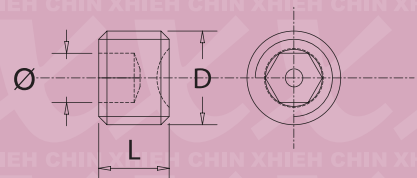
A1005 D*L*Ø
