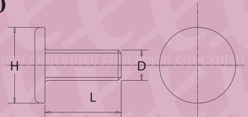
A1040 D*L*H
